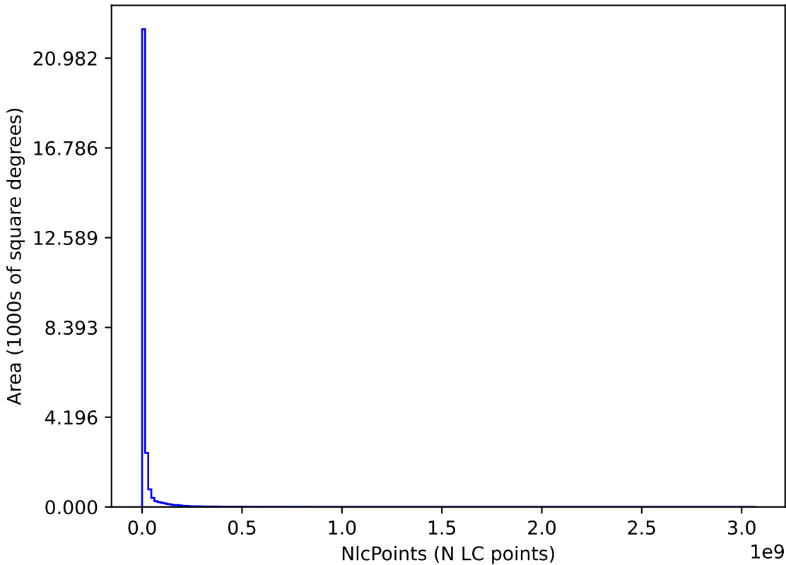
no_long_daily_v3.4_10yrs : NlcPoints
