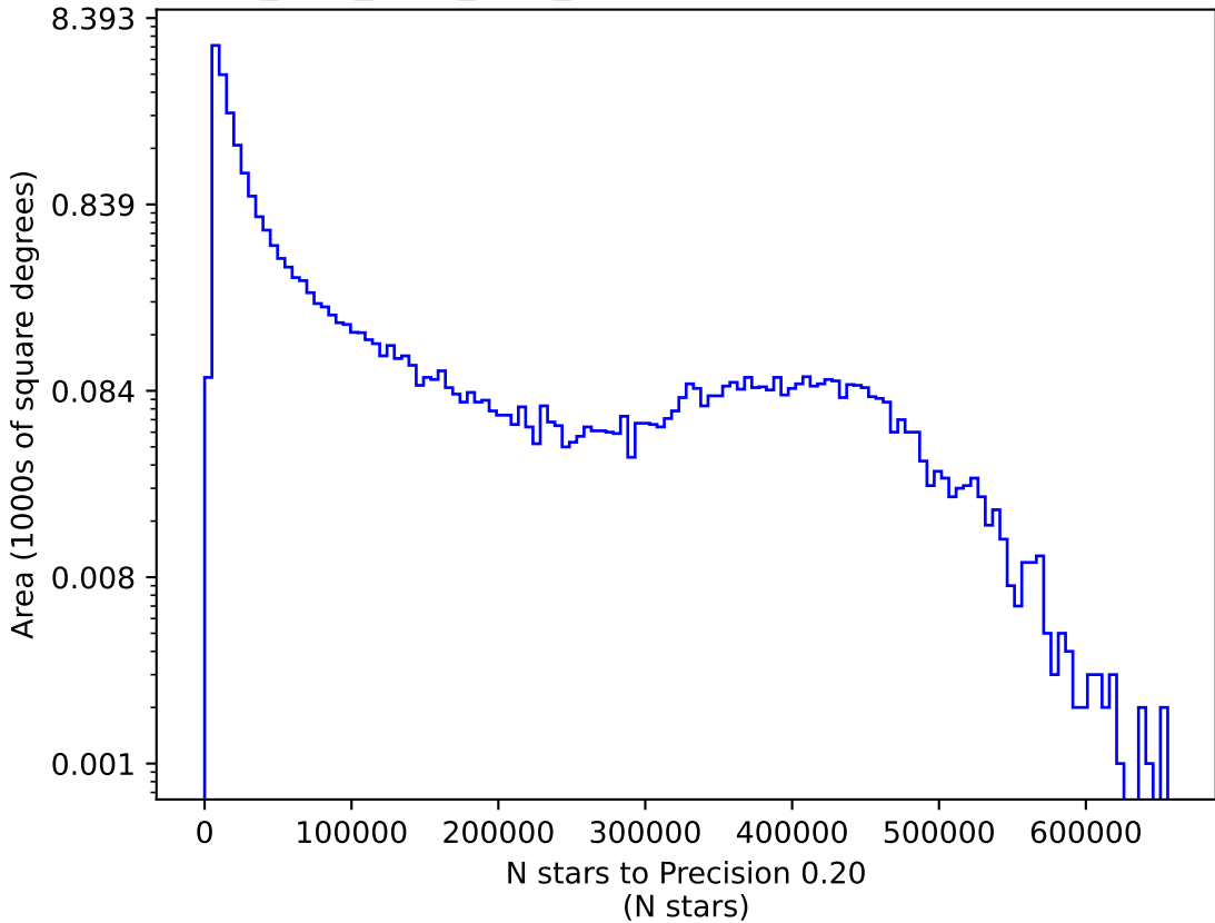
no_long_daily_v3.4_10yrs z: N stars to Precision 0.20
