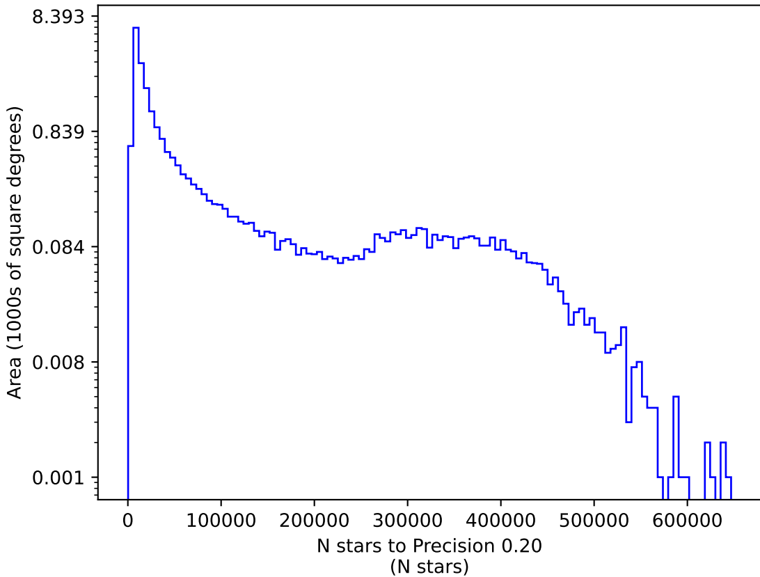
no_long_daily_v3.4_10yrs y: N stars to Precision 0.20
