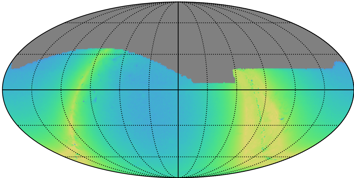
no_long_daily_v3.4_10yrs r: N stars to Precision 0.20
