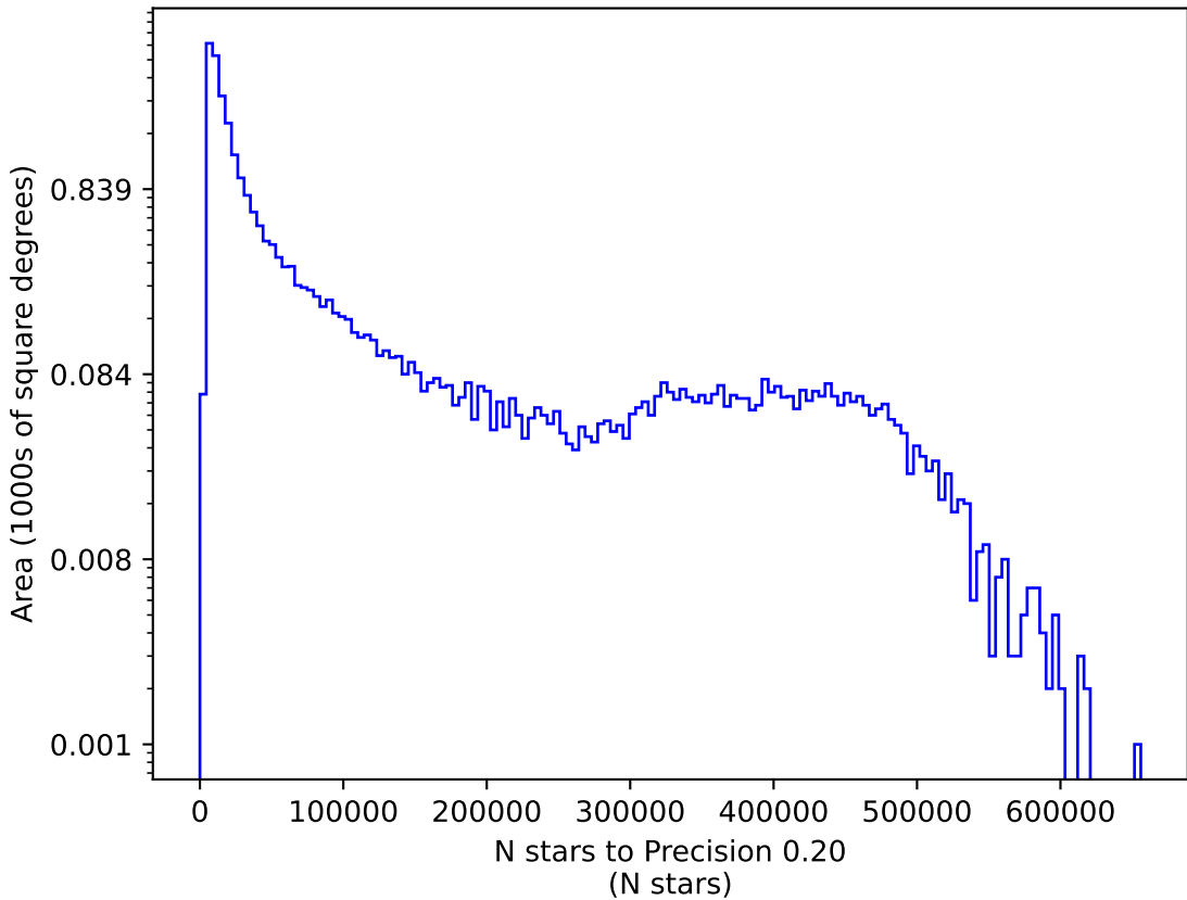
no_long_daily_v3.4_10yrs r: N stars to Precision 0.20
