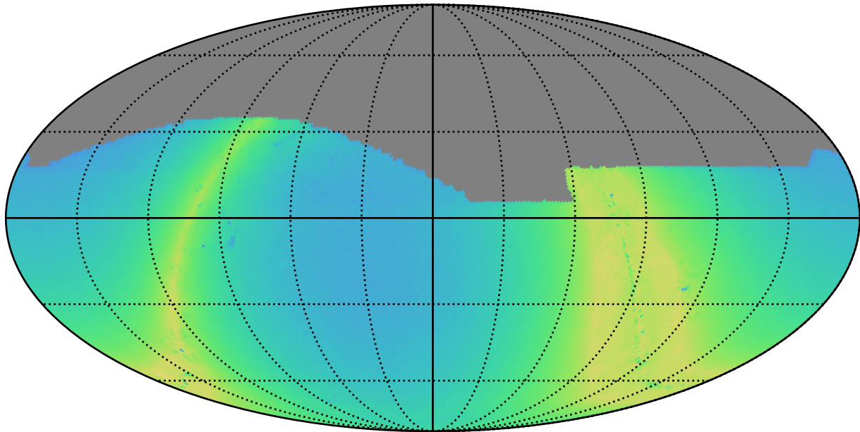
no_long_daily_v3.4_10yrs i: N stars to Precision 0.20
