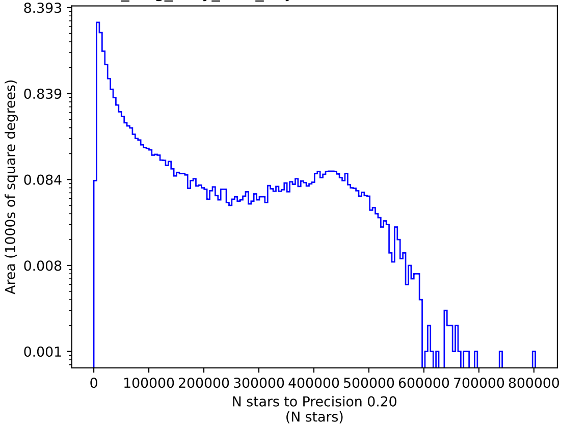
no_long_daily_v3.4_10yrs i: N stars to Precision 0.20
