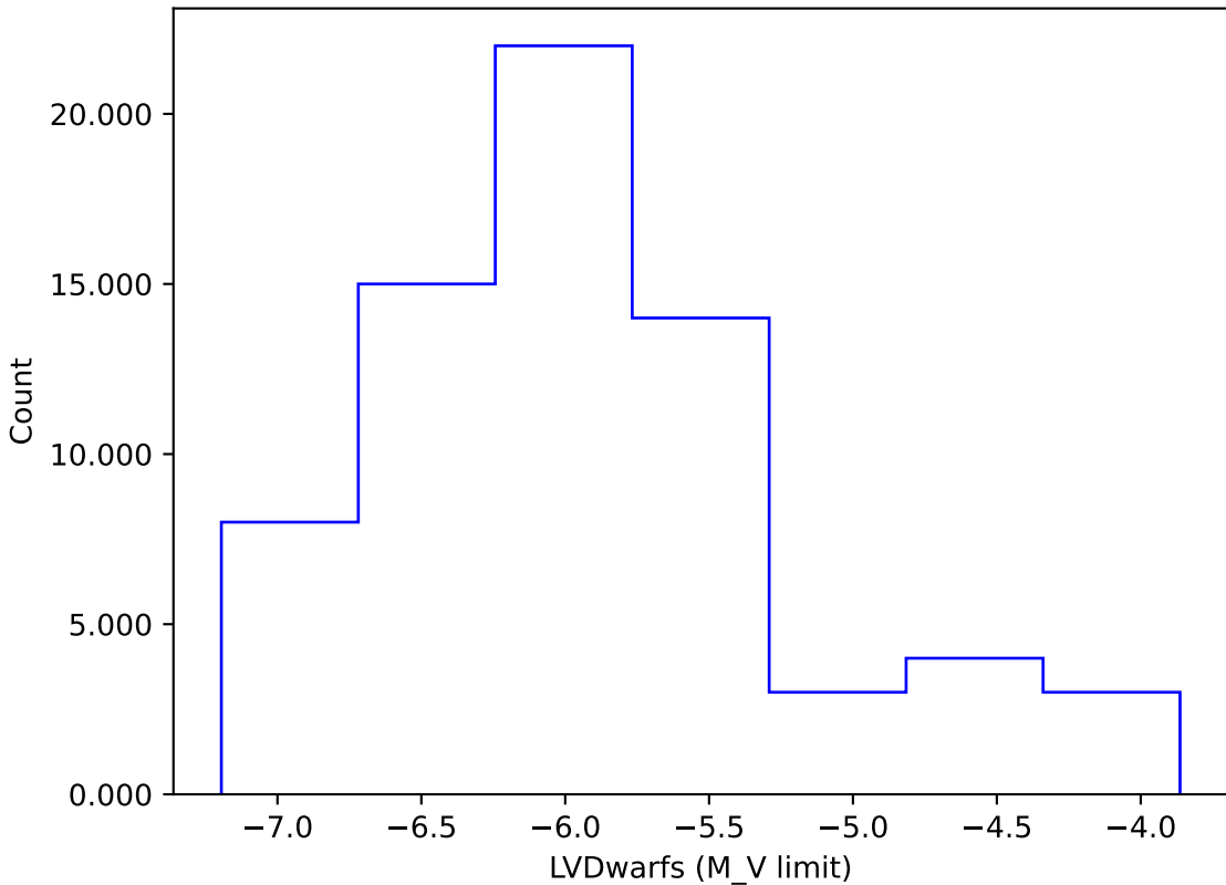
no_long_daily_v3.4_10yrs gi: LVDwarfs
