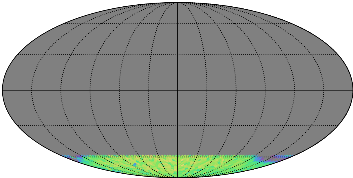
no_long_daily_v3.4_10yrs gi SCP: LVDwarfs
