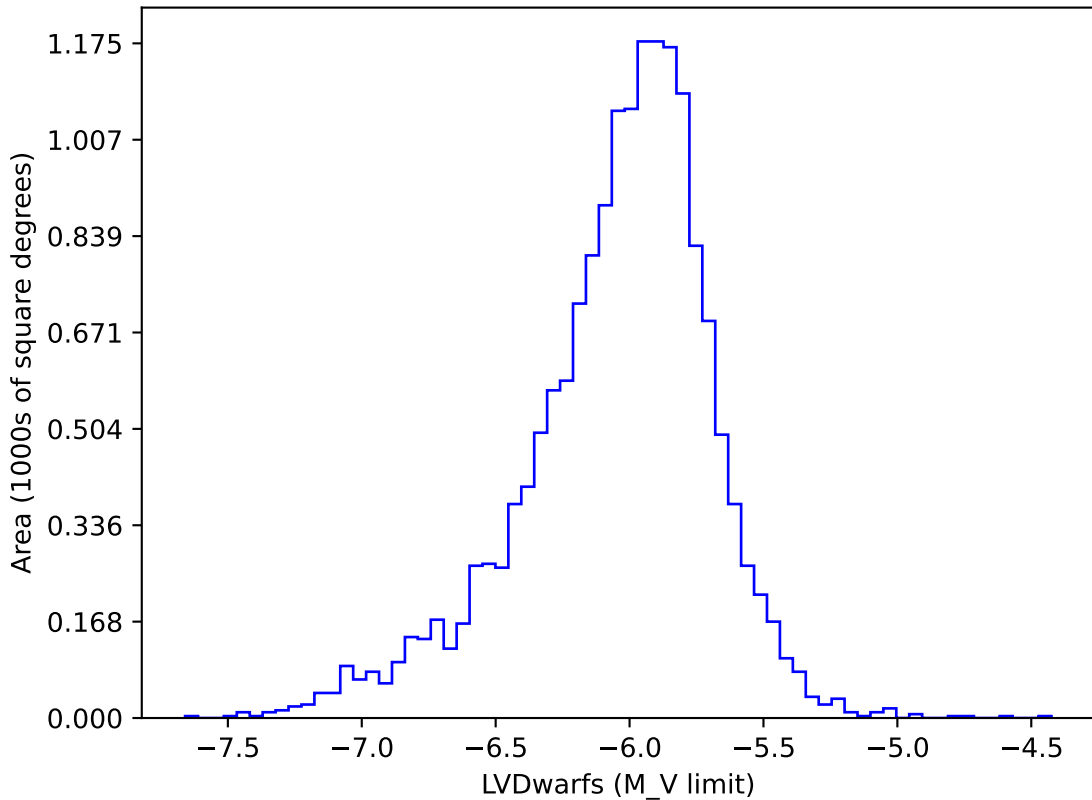
no_long_daily_v3.4_10yrs gi: LVDwarfs
