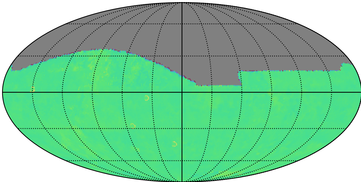
no_long_daily_v3.4_10yrs z: Kuiper rotTelPos
