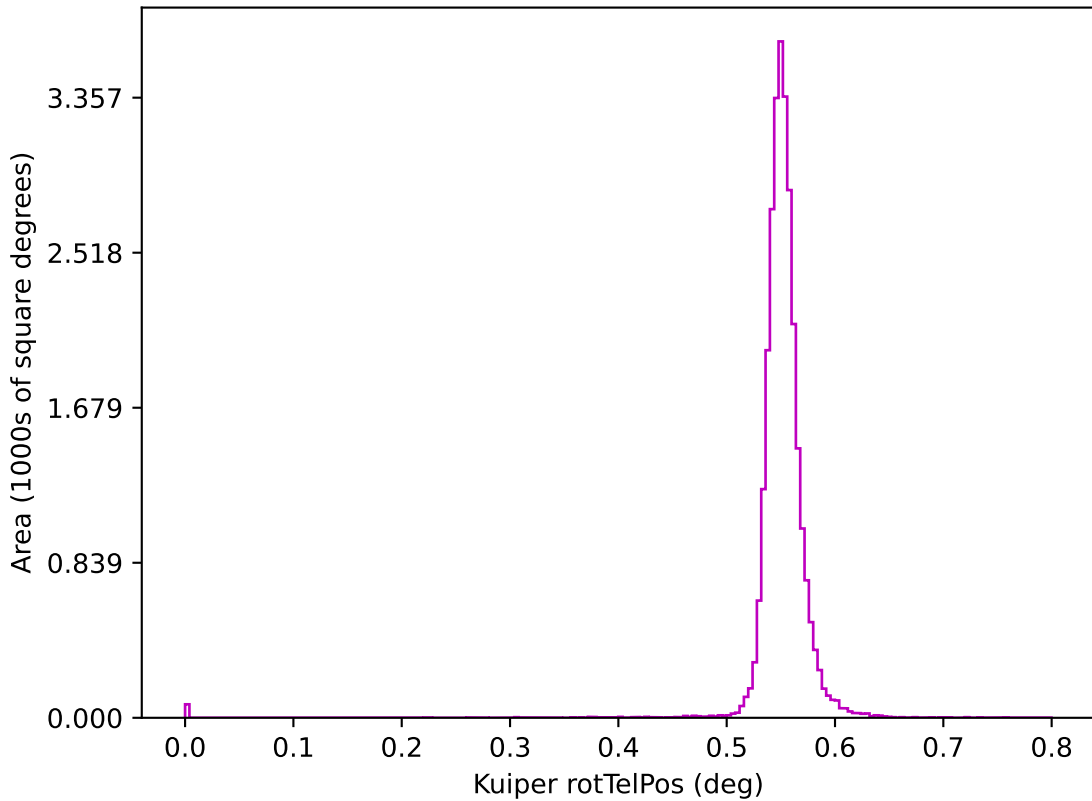
no_long_daily_v3.4_10yrs z: Kuiper rotTelPos
