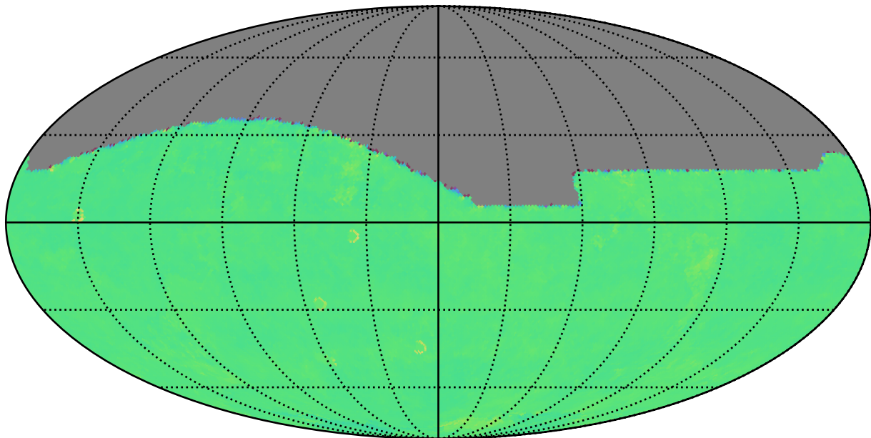
no_long_daily_v3.4_10yrs r: Kuiper rotTelPos
