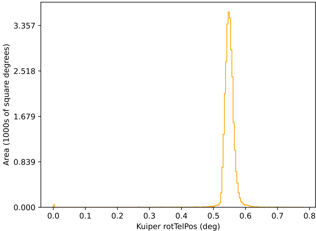
no_long_daily_v3.4_10yrs r: Kuiper rotTelPos
