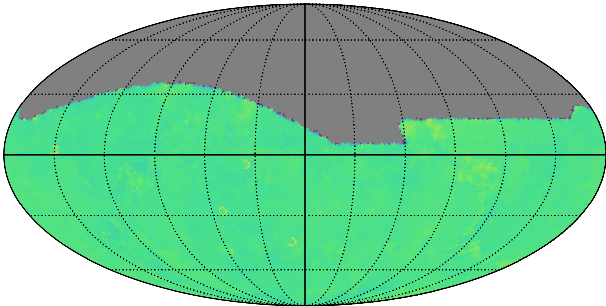
no_long_daily_v3.4_10yrs g: Kuiper rotTelPos
