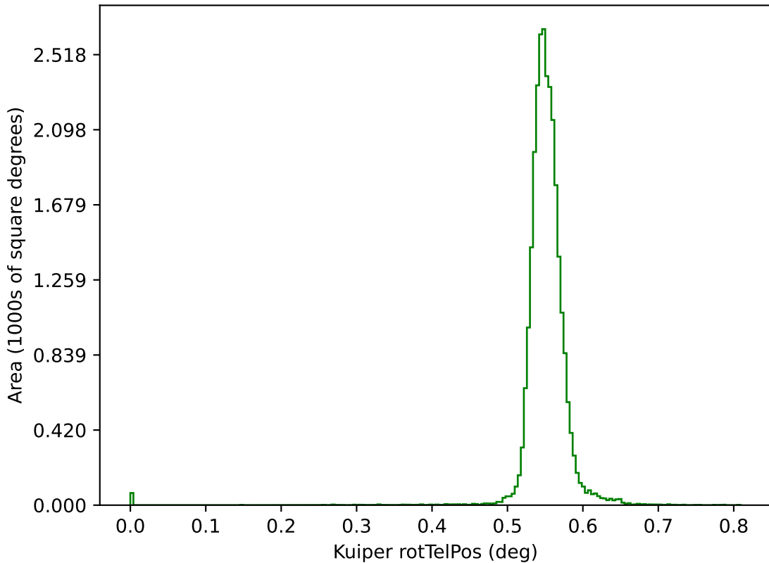
no_long_daily_v3.4_10yrs g: Kuiper rotTelPos
