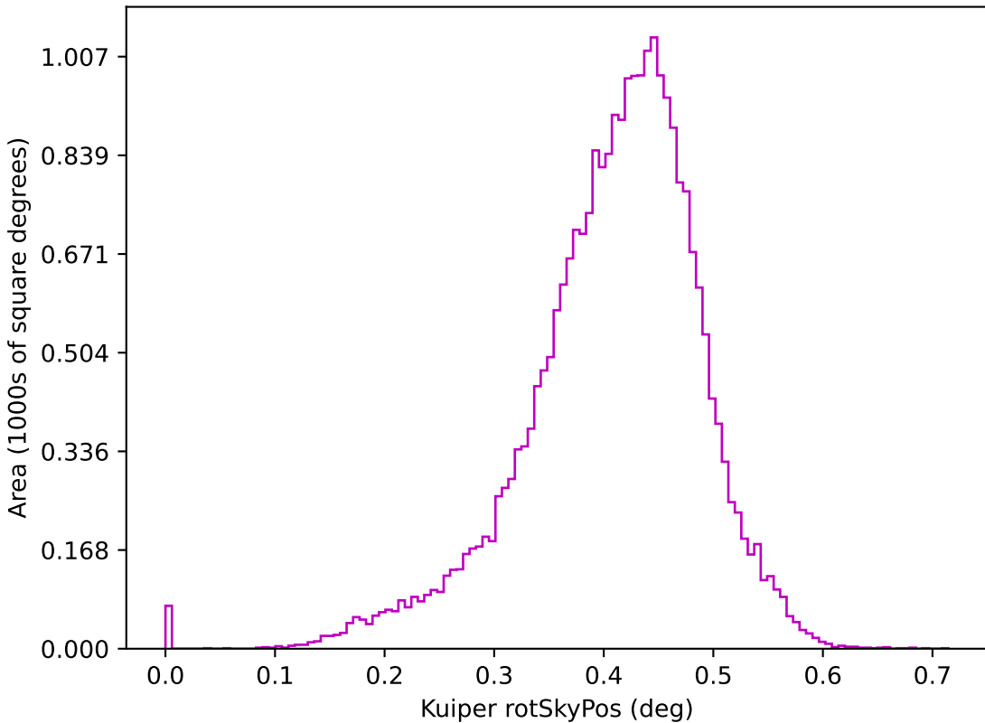
no_long_daily_v3.4_10yrs z: Kuiper rotSkyPos
