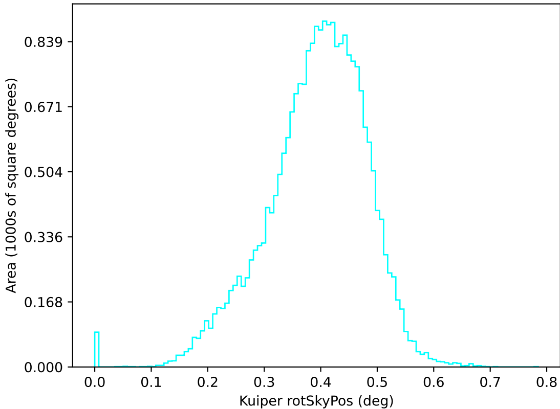
no_long_daily_v3.4_10yrs u: Kuiper rotSkyPos
