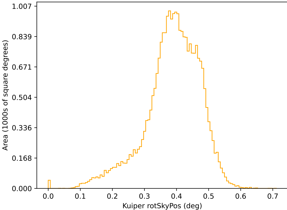
no_long_daily_v3.4_10yrs r: Kuiper rotSkyPos
