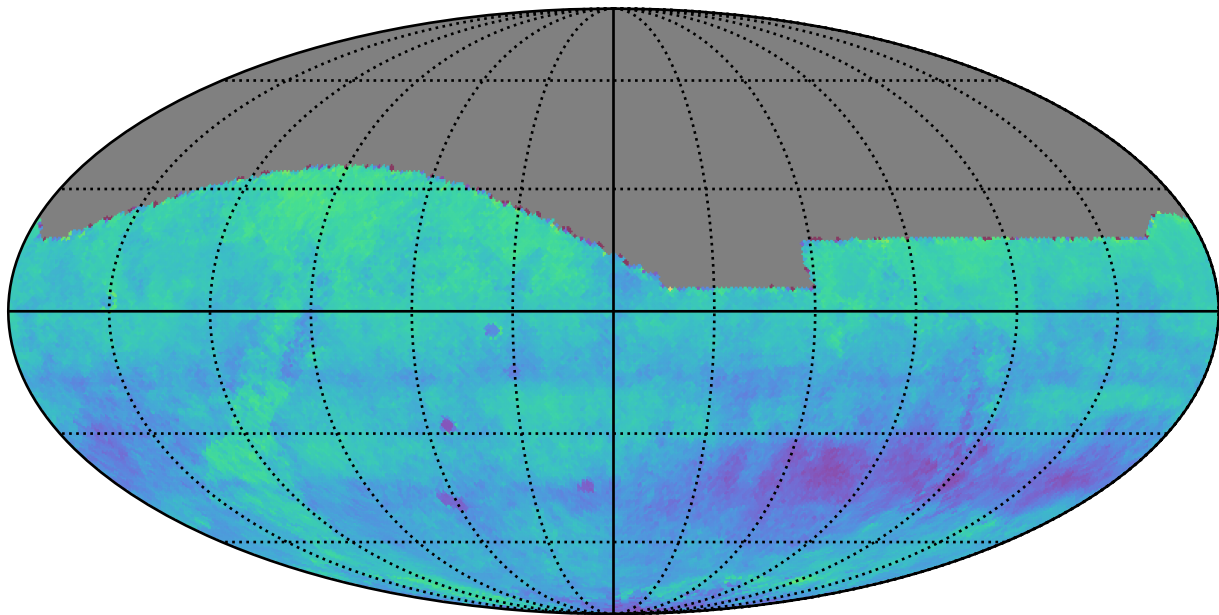
no_long_daily_v3.4_10yrs i: Kuiper rotSkyPos
