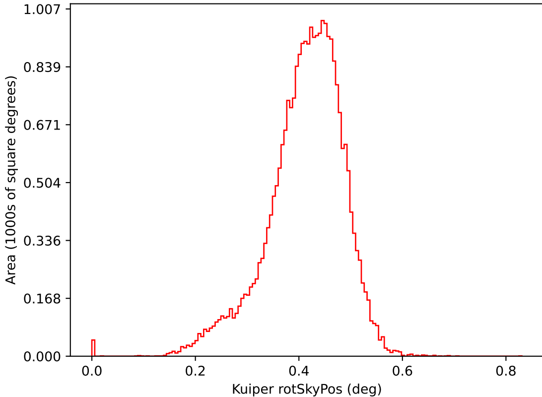
no_long_daily_v3.4_10yrs i: Kuiper rotSkyPos
