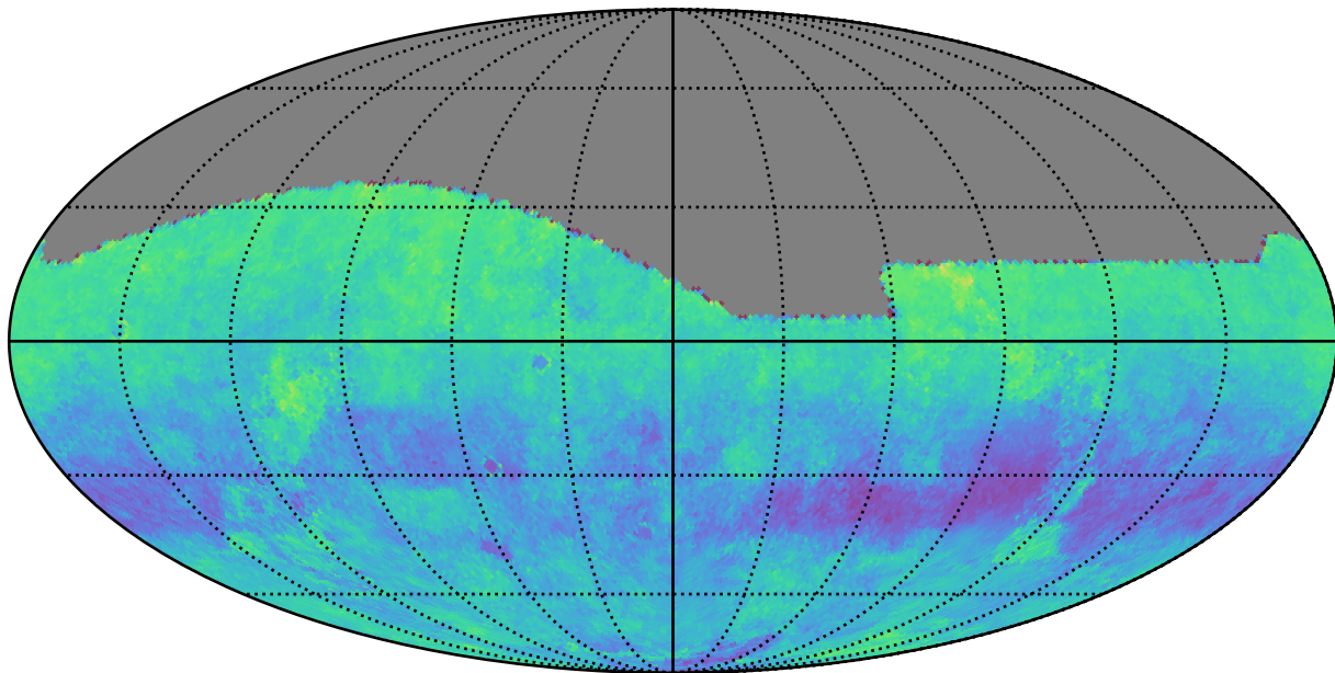
no_long_daily_v3.4_10yrs g: Kuiper rotSkyPos
