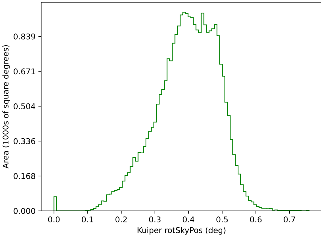
no_long_daily_v3.4_10yrs g: Kuiper rotSkyPos
