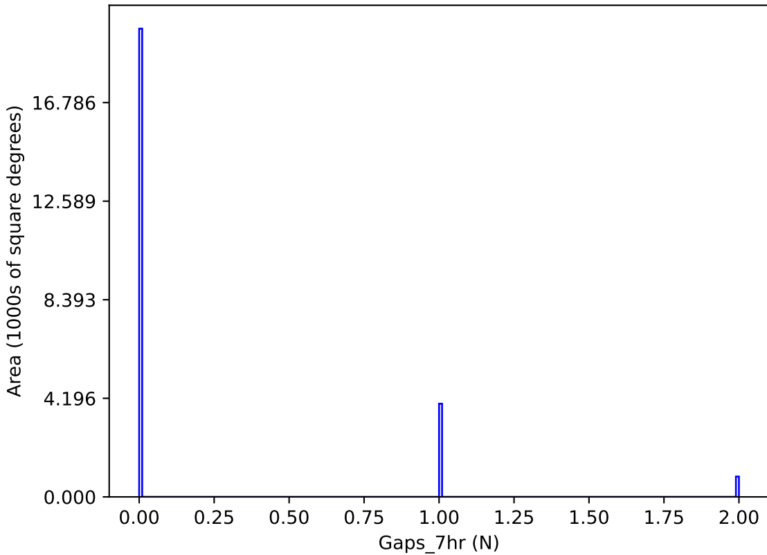
no_long_daily_v3.4_10yrs y band: Gaps_7hr
