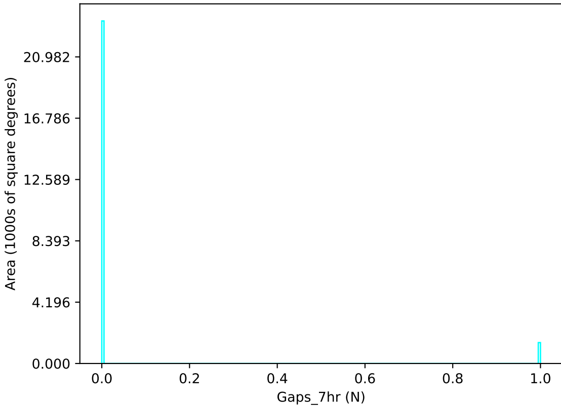
no_long_daily_v3.4_10yrs u band: Gaps_7hr
