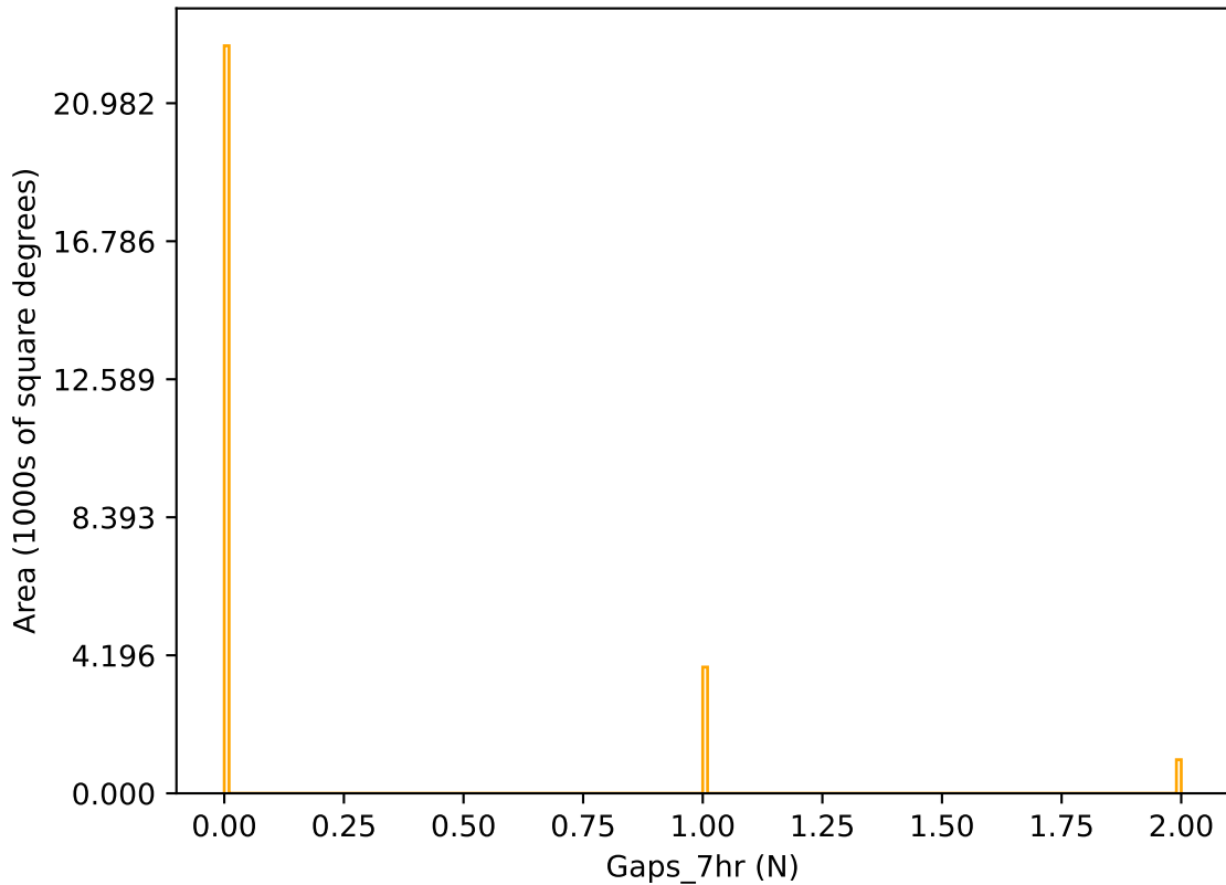
no_long_daily_v3.4_10yrs r band: Gaps_7hr
