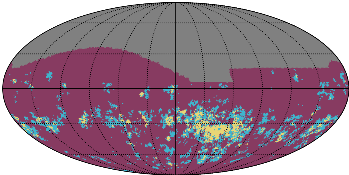
no_long_daily_v3.4_10yrs i band: Gaps_7hr
