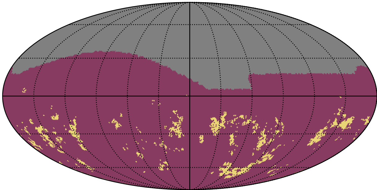
no_long_daily_v3.4_10yrs g band: Gaps_7hr
