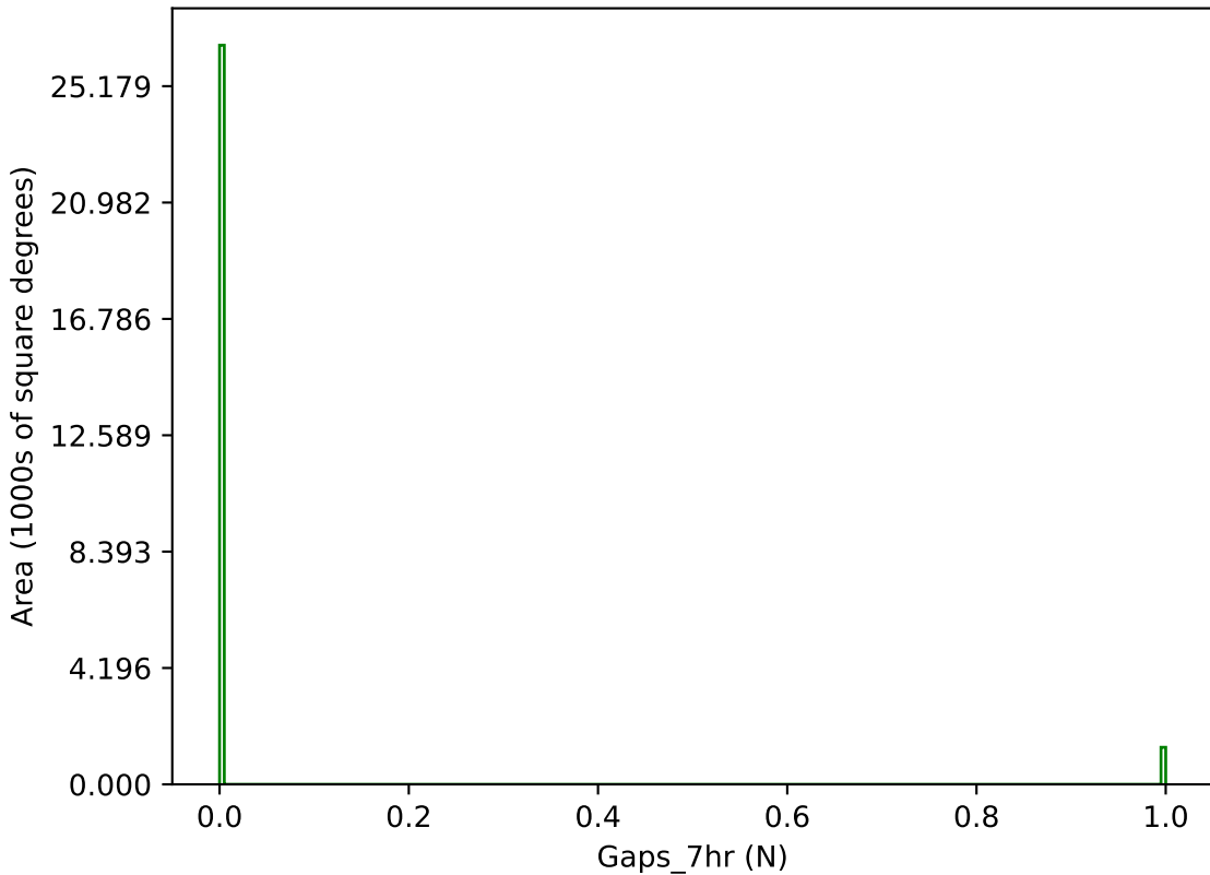
no_long_daily_v3.4_10yrs g band: Gaps_7hr
