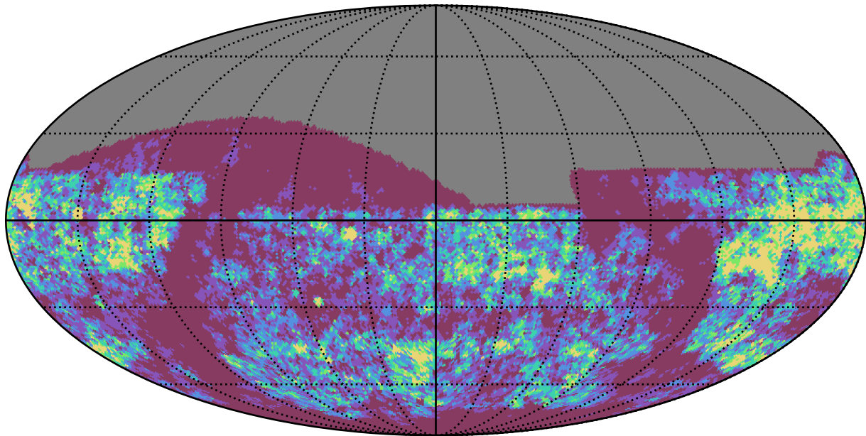
no_long_daily_v3.4_10yrs z band: Gaps_3hr
