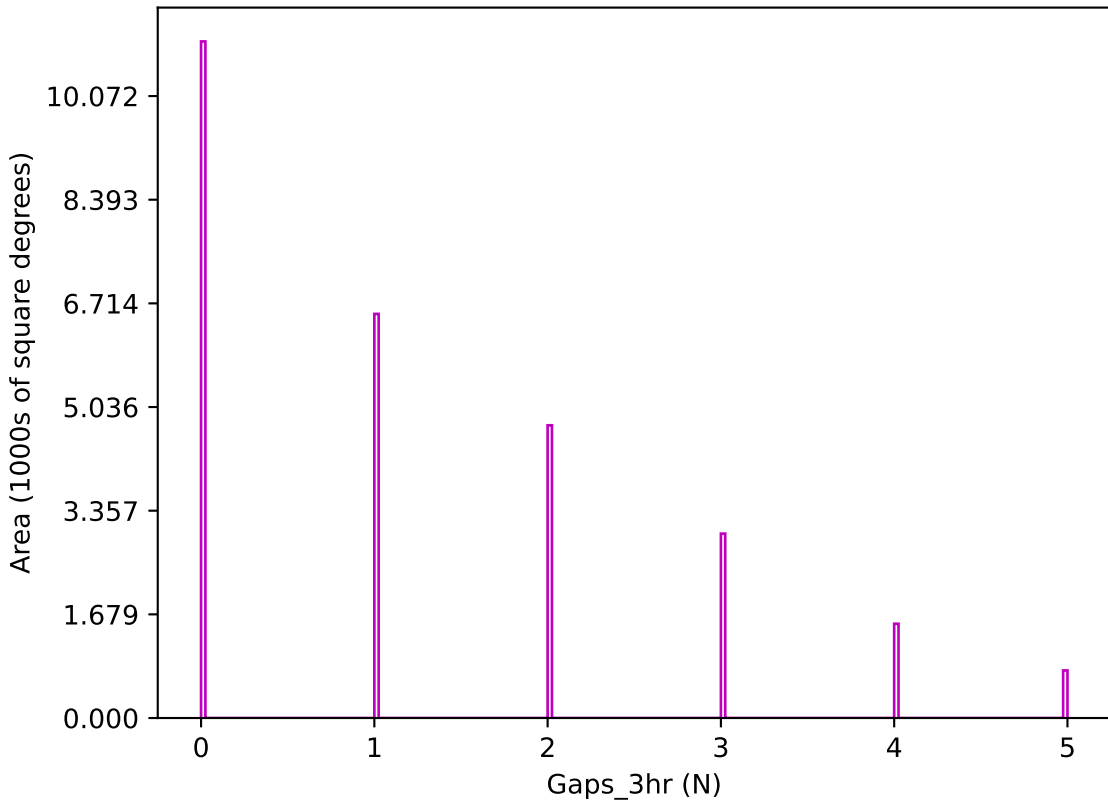
no_long_daily_v3.4_10yrs z band: Gaps_3hr
