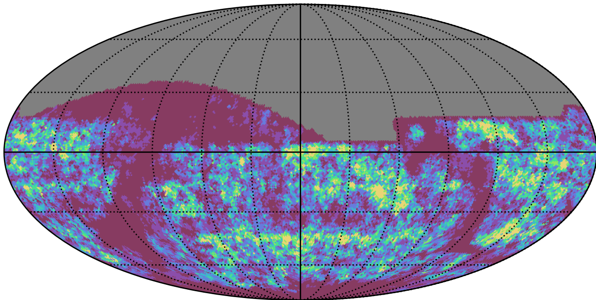
no_long_daily_v3.4_10yrs r band: Gaps_3hr
