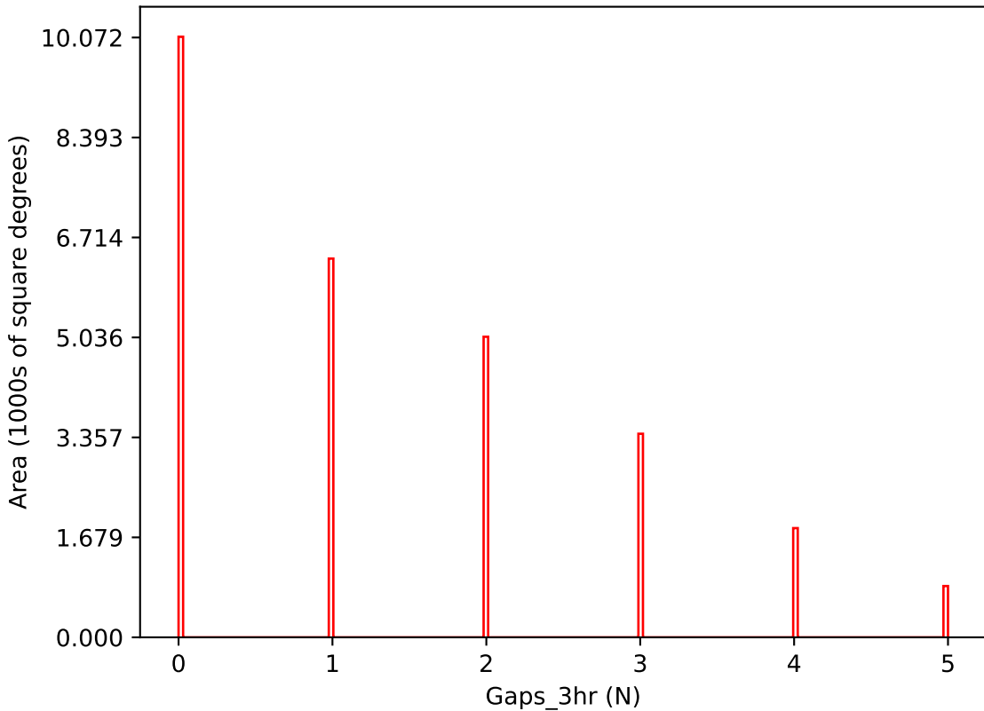
no_long_daily_v3.4_10yrs i band: Gaps_3hr
