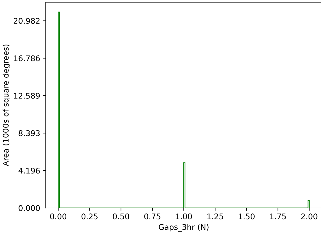
no_long_daily_v3.4_10yrs g band: Gaps_3hr
