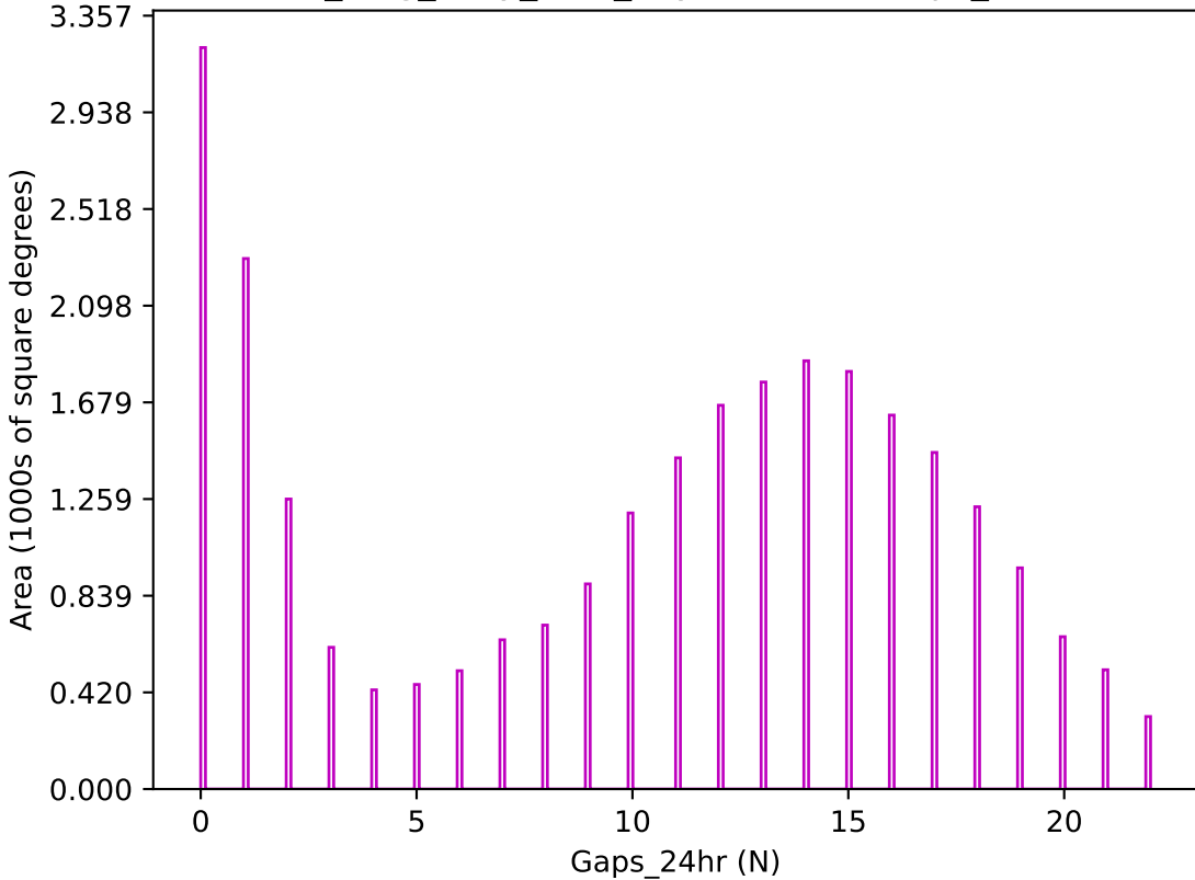
no_long_daily_v3.4_10yrs z band: Gaps_24hr
