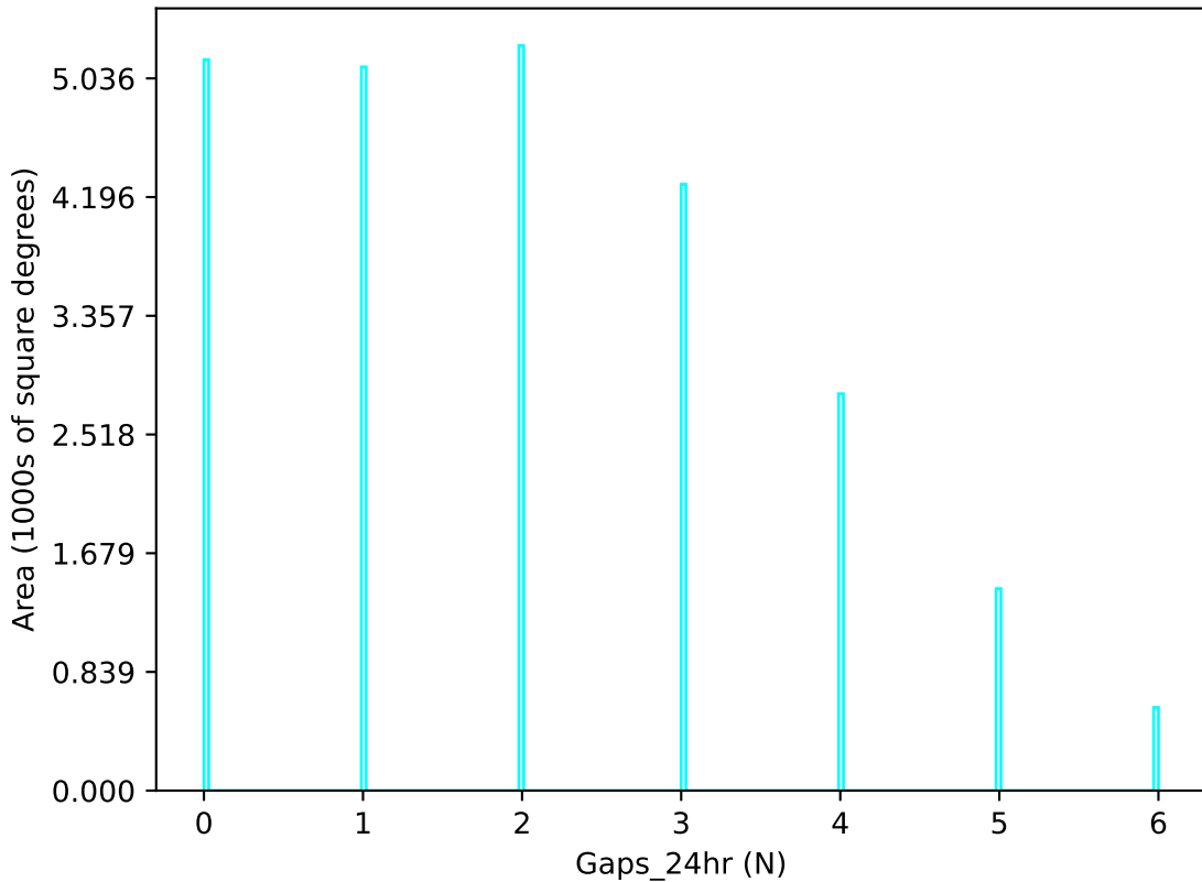
no_long_daily_v3.4_10yrs u band: Gaps_24hr
