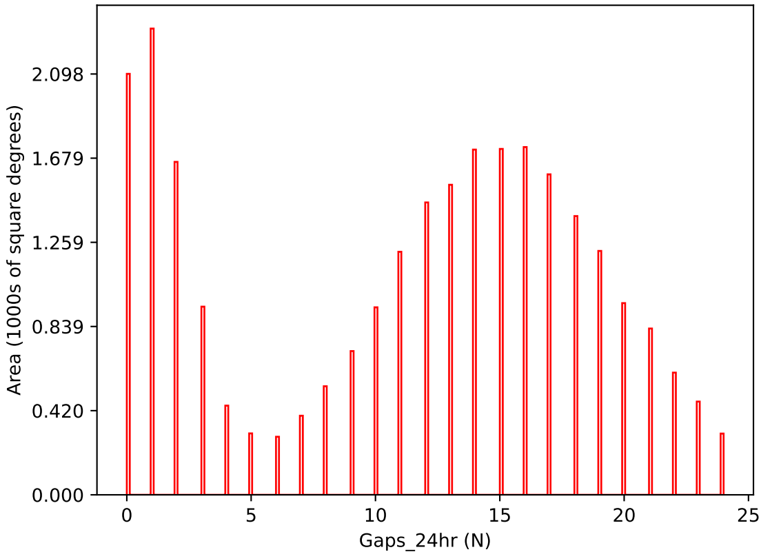
no_long_daily_v3.4_10yrs i band: Gaps_24hr
