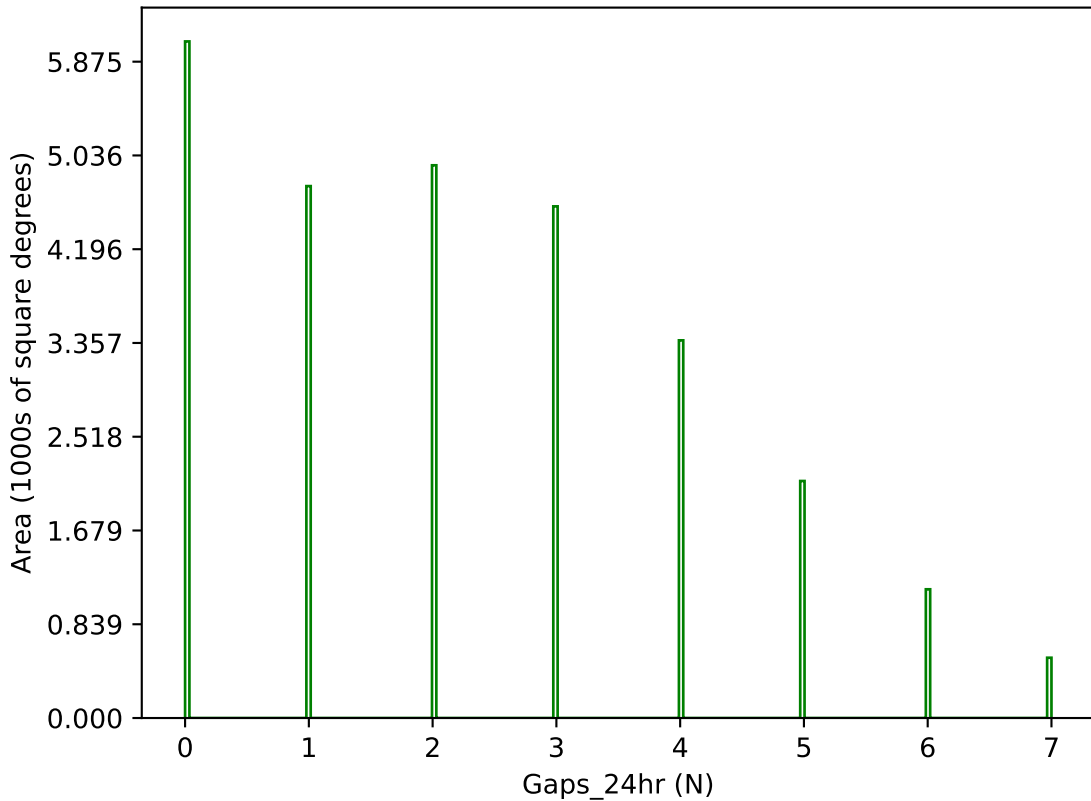
no_long_daily_v3.4_10yrs g band: Gaps_24hr
