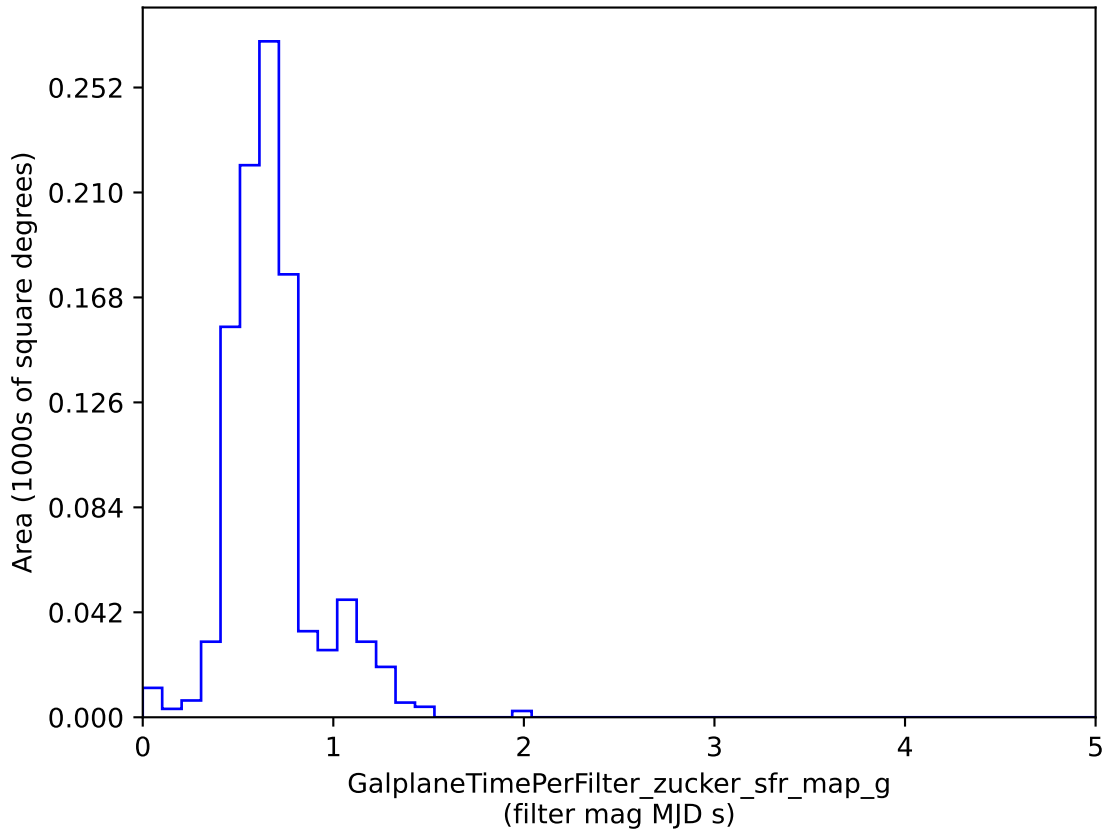
no_long_daily_v3.4_10yrs : GalplaneTimePerFilter_zucker_sfr_map_g
