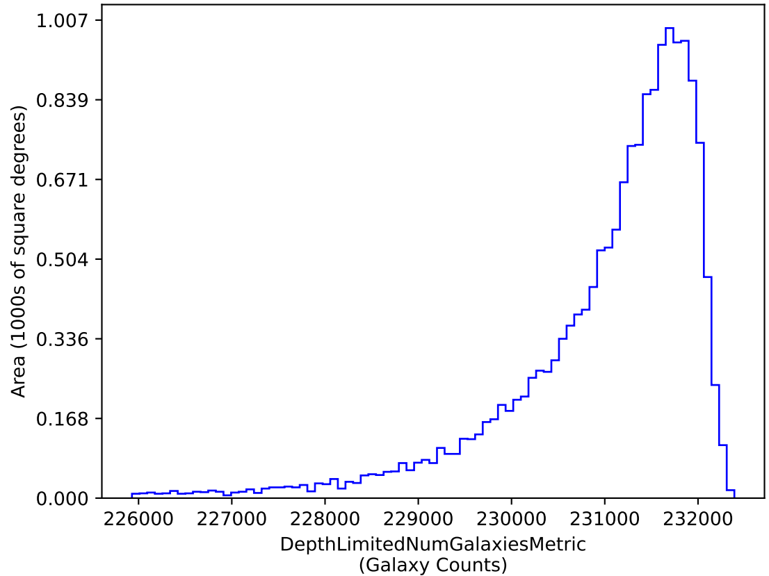
no_long_daily_v3.4_10yrs i band galaxies non-DD: DepthLimitedNumGalaxiesMetric
