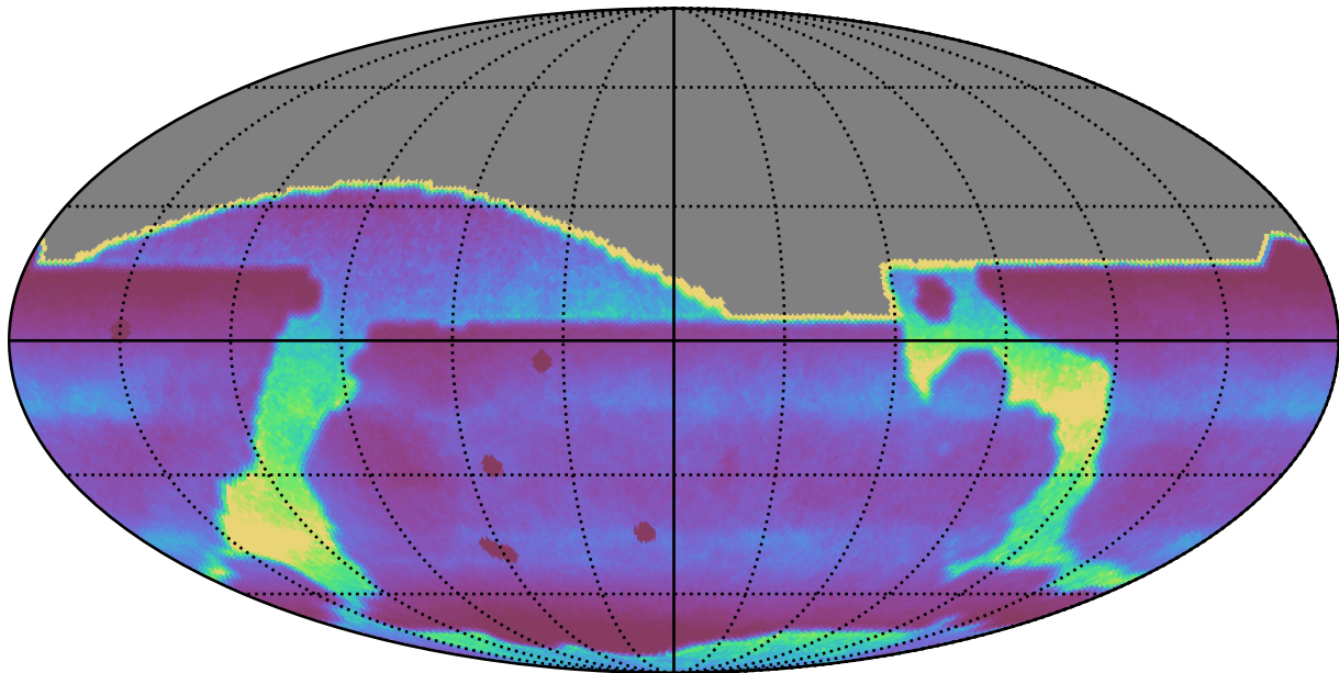
no_long_daily_v3.4_10yrs : DCRprecision
