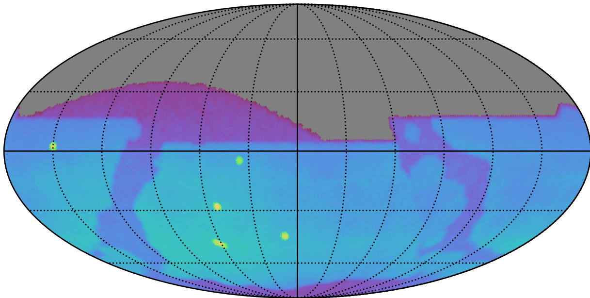
no_long_daily_v3.4_10yrs : Brown Dwarf, L7
