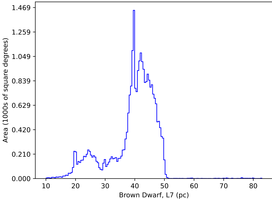
no_long_daily_v3.4_10yrs : Brown Dwarf, L7
