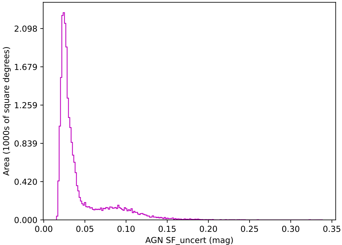
no_long_daily_v3.4_10yrs z band: AGN SF_uncert
