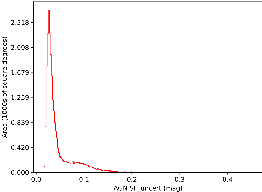
no_long_daily_v3.4_10yrs i band: AGN SF_uncert
