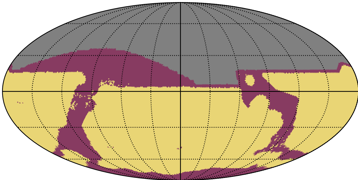
no_long_daily_v3.4_10yrs All sky: RapidRevisits
