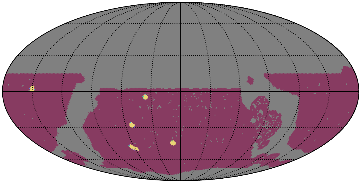
no_long_daily_v3.4_10yrs WFD: NumberOfQuickRevisits
