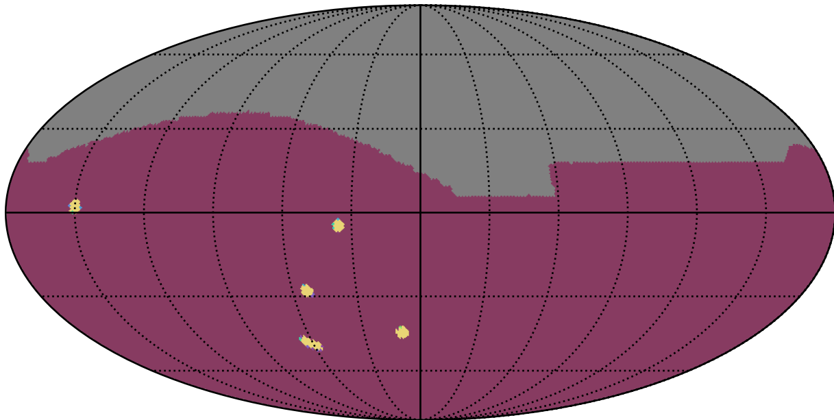
no_long_daily_v3.4_10yrs All sky: NumberOfQuickRevisits
