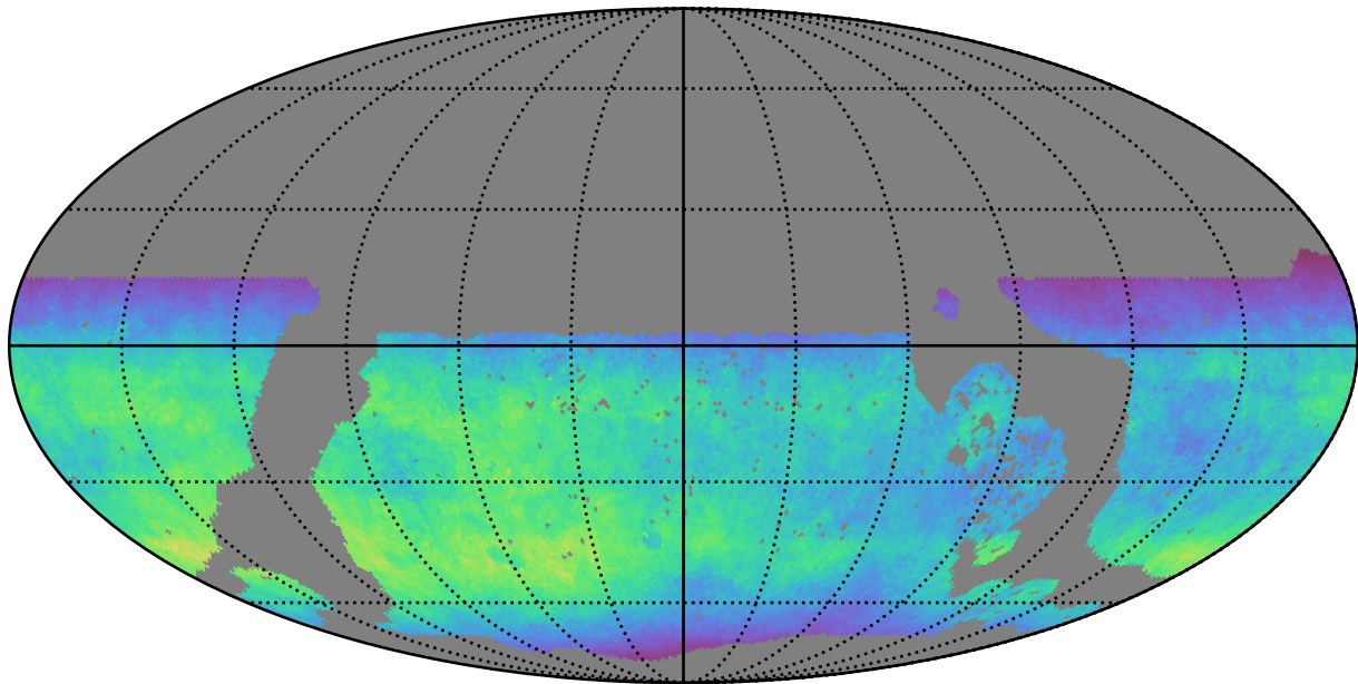
no_long_daily_v3.4_10yrs WFD y band: Normalized Teff
