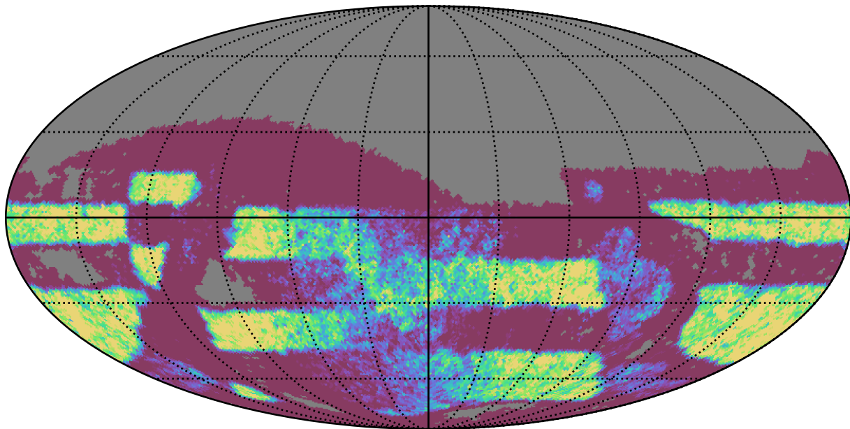
no_long_daily_v3.4_10yrs Yr 3-4 z band: NVisits
